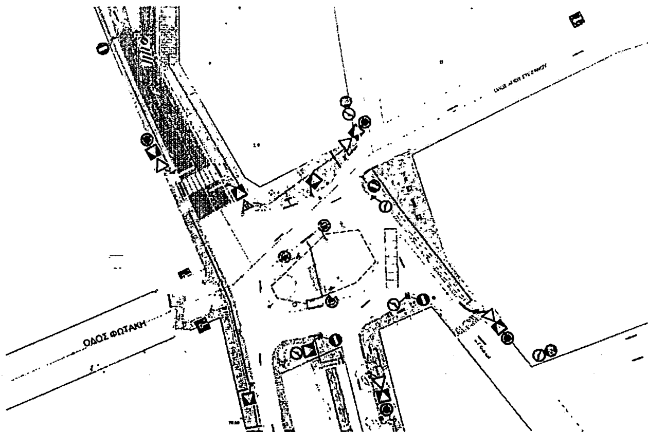
Εικόνα 20. διαμόρφωση έργου με προβλέψεις κυκλοφορίας και σήμανσης - περιοχή 10
