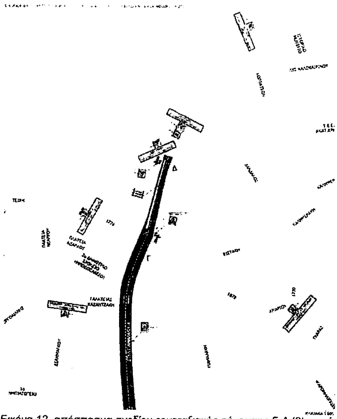
Εικόνα 12. απόσπασμα σχεδίου εργοταξιακής σήμανσης Γ-Δ (2)_επίσταση στη ζώνη έργων
