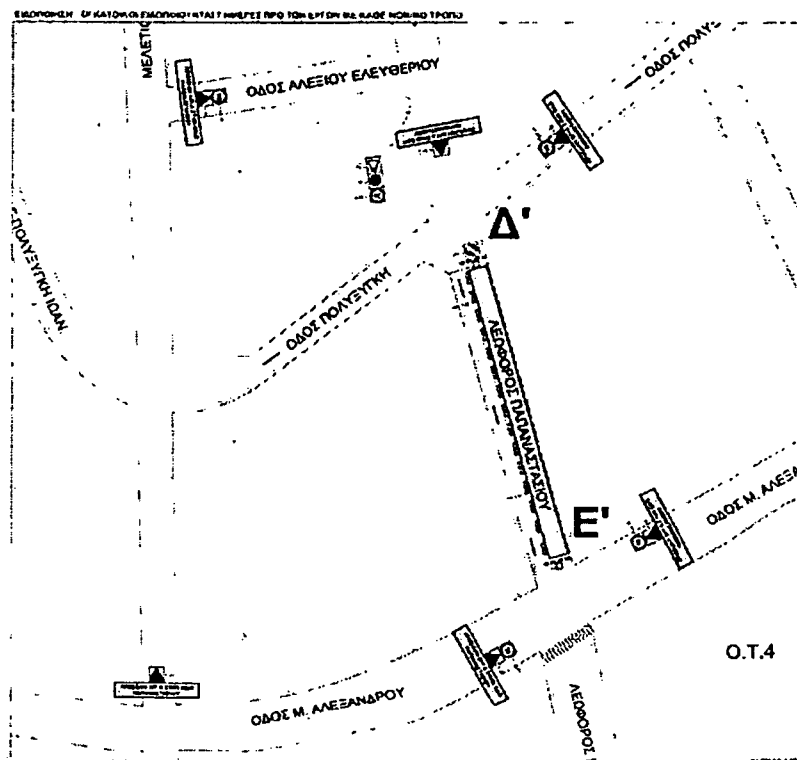
Εικόνα 12. απόσπασμα σχεδίου εργοταξιακής σήμανσης Δ'-Ε'_ εστίαση στη ζώνη έργων
