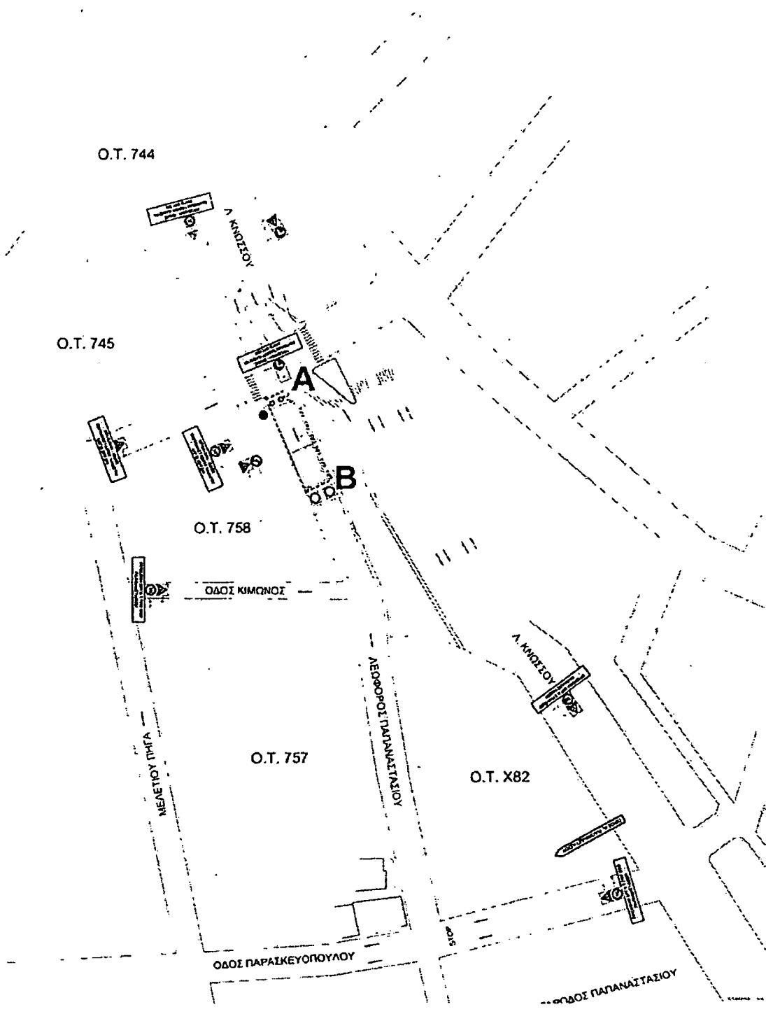
Εικόνα 5. απόσπασμα σχεδίου εργοταξιακής σήμανσης Α-Β_ εστίαση στη ζώνη έργων
