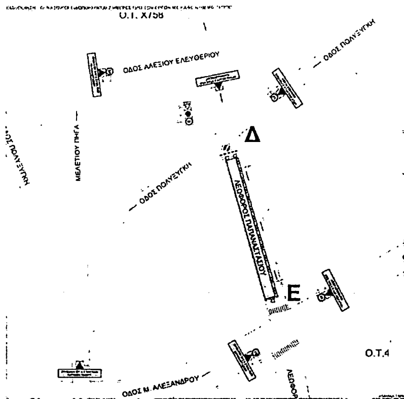
Εικόνα 11. απόσπασμα σχεδίου εργοταξιακής σήμανσης Δ-Ε_ εστίαση στη ζώνη έργων
