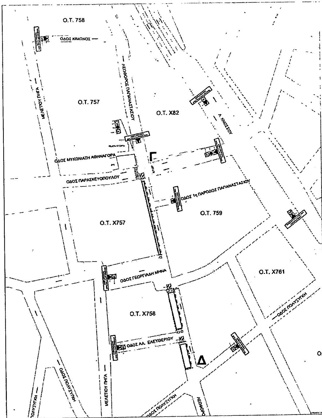
Εικόνα 9. απόσπασμα σχεδίου εργαταξιακής σήμανσης Γ-Δ_ εστίαση στη ζώνη έργων
