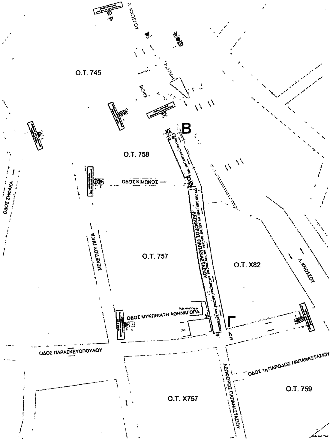
Εικόνα 7. απόσπασμα σχεδίου εργοταξιακής σήμανσης Β-Γ_ εστίαση στη ζώνη έργων
