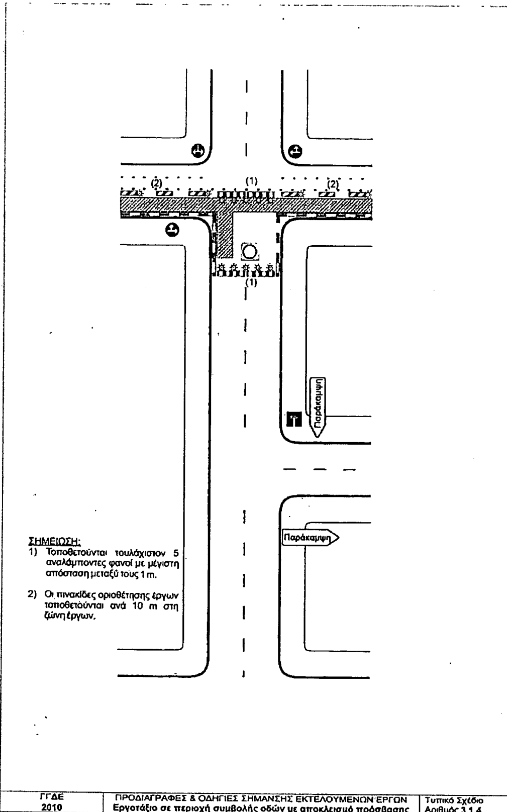
Εικόνα 3. τυπικό σχέδιο Αρ. 3.1.4 «Εργοτάξιο σε περιοχή συμβολής οδών με αποκλεισμό πρόσβασης», κατά ΟΜΟΕ ΣΕΕΟ ΦΕΚ 905/Β/2011 (ΔΜΕΟ/Ο/613/2011) – εφαρμογή στο τμήμα Α-Β
