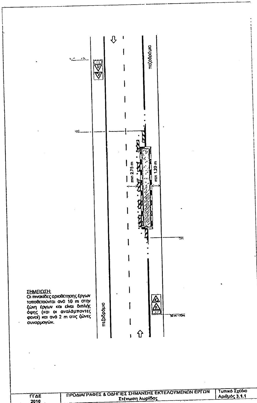
Εικόνα 4. τυπικό σχέδιο Αρ. 3.1.1 «Στένωση λωρίδας», κατά ΟΜΟΕ ΣΕΕΟ ΦΕΚ 905/Β/2011 (ΔΜΕΟ/Ο/613/2011) - εφαρμογή στα τμήματα Β-Γ, Γ-Δ, Δ-Ε, Δ'-Ε', Ε-Ζ
