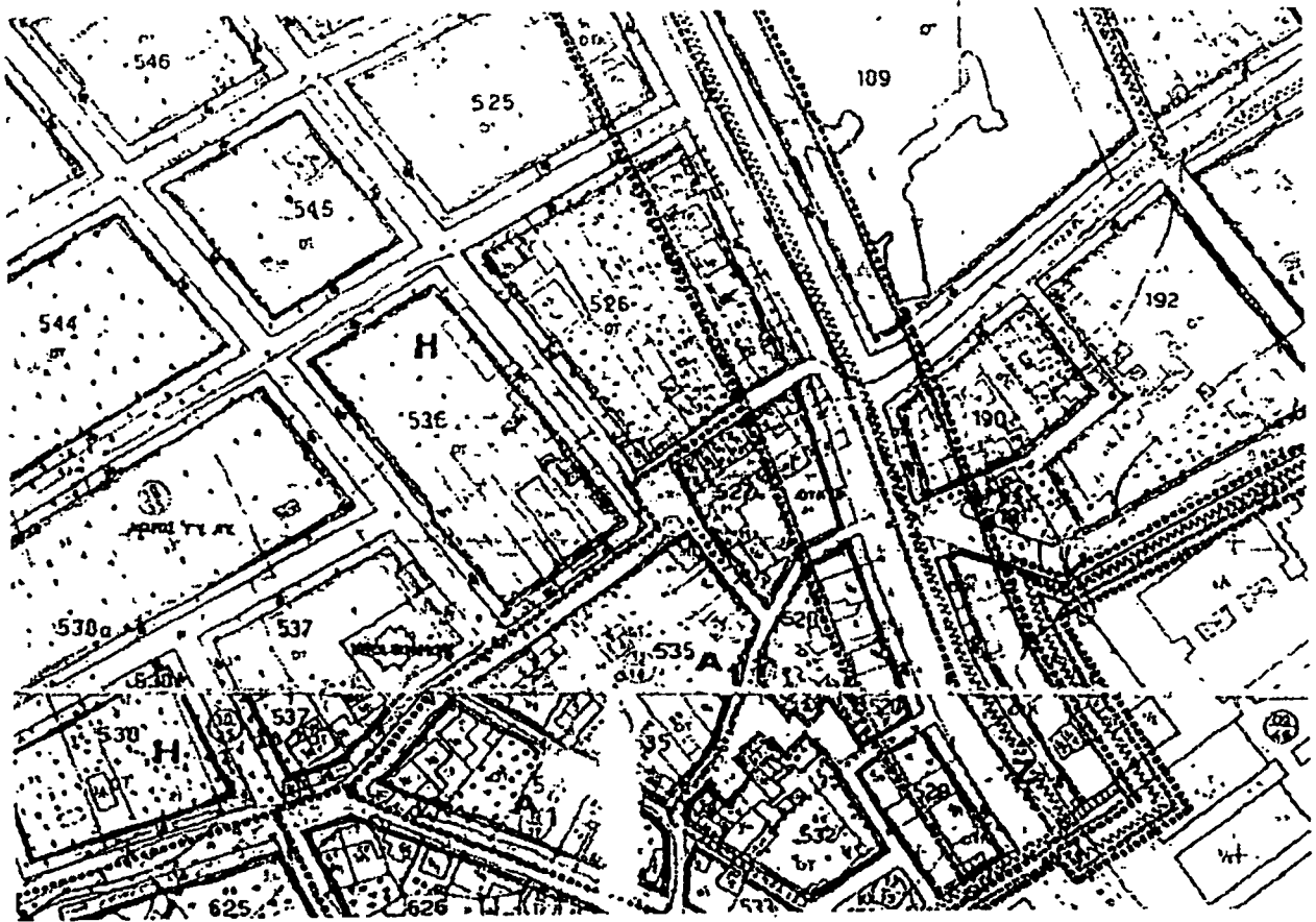
ΕΙΚΟΝΑ 1.ΙΣΧΥΟΝ ΡΥΜΟΤΟΜΙΚΟ ΣΧΕΔΙΟ
